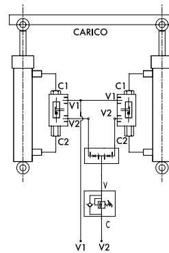
SCHEMA DI MONTAGGIO MOUNTING DIAGRAM
