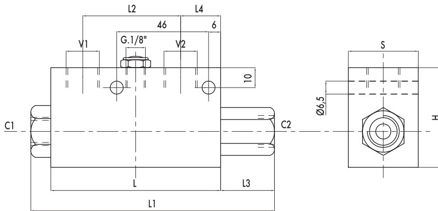
SCHEMA DI MONTAGGIO MOUNTING DIAGRAM
